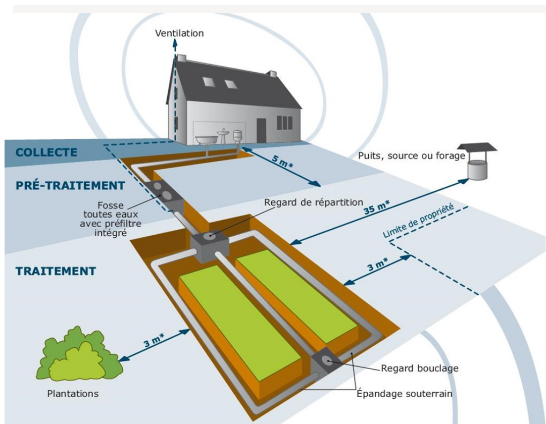
Schéma du fonctionnement d'une installation d'assainissement non collectif d'un logement individuel
